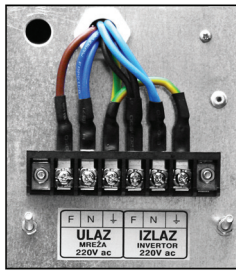
Izgled priključne kutije sa rasporedom klem
